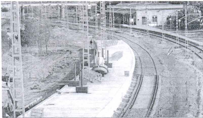
Imagen reciente de las obras de Alta Velocidad que se ejecutan a su paso por la estación puertorealense.
